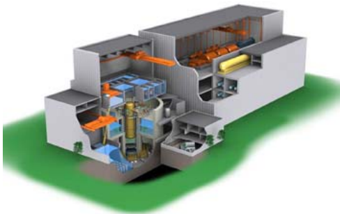
ESBWR
